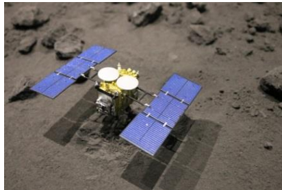
小惑星リュウグウ模擬地形
